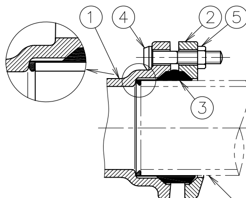
継手各部の名称
