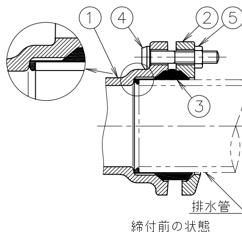
継手各部の名称
