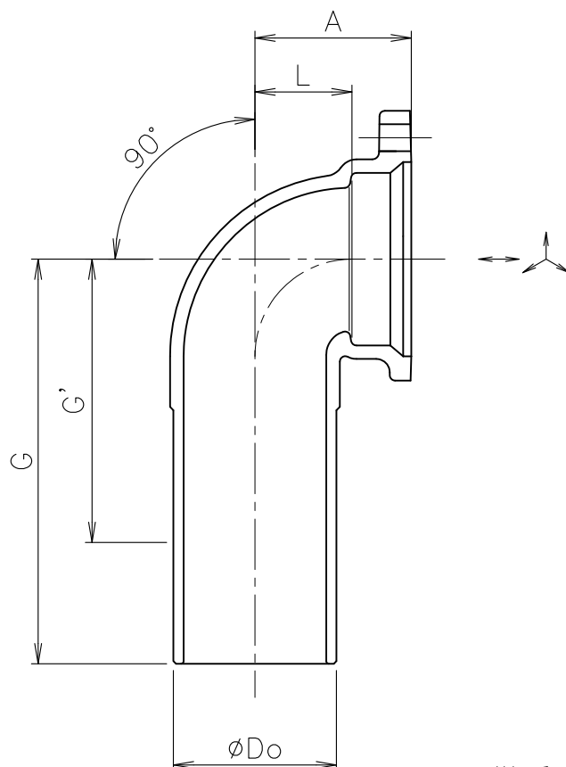
継手各部の名称
