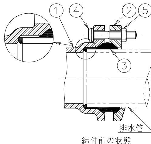
継手各部の名称 締付後の状態
