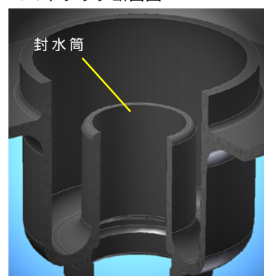
c. トラップ断面図
