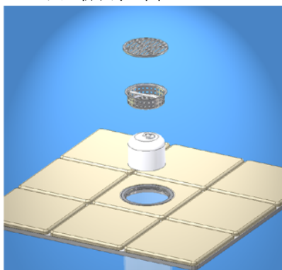
b. ワン取り外し図
