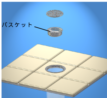
a. バスケット取り外し図
