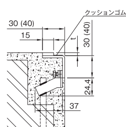
ピットふた用 CA-Q 枠定価表 (L40・長さ 0.5m・四方枠)
