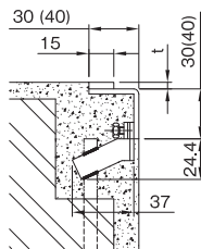
ピットふた用 CA 枠定価表 (L40・長さ 0.5m・四方枠)
