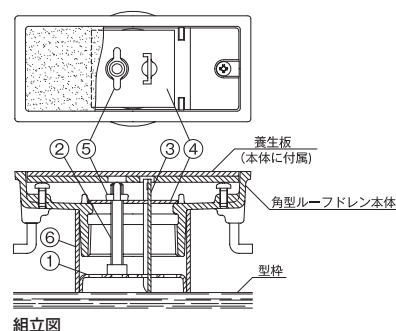
組立図
