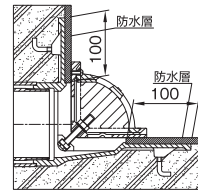
防水層張掛け幅
