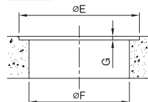
取付穴寸法
