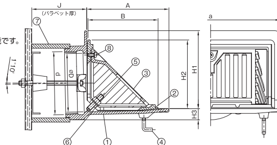
排水器具
