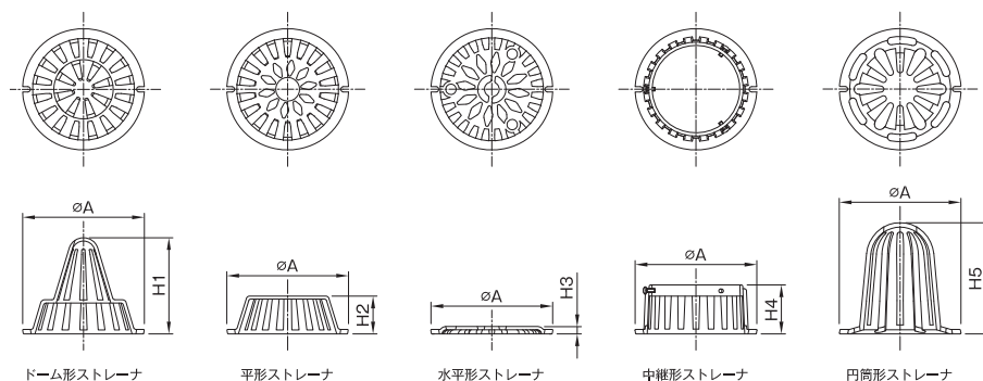
寸法表 (mm)
