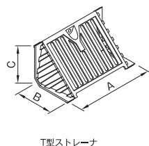
寸法表 (mm)
