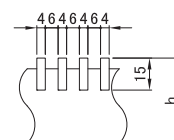
グレーチング蓋ピン詳細図
