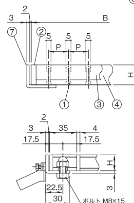
ボルト固定部詳細
