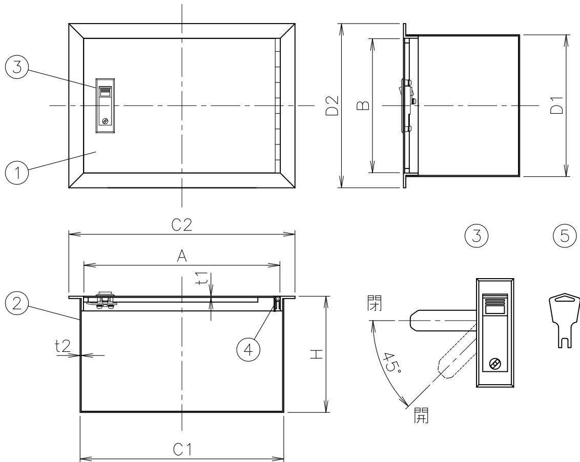
寸法表
