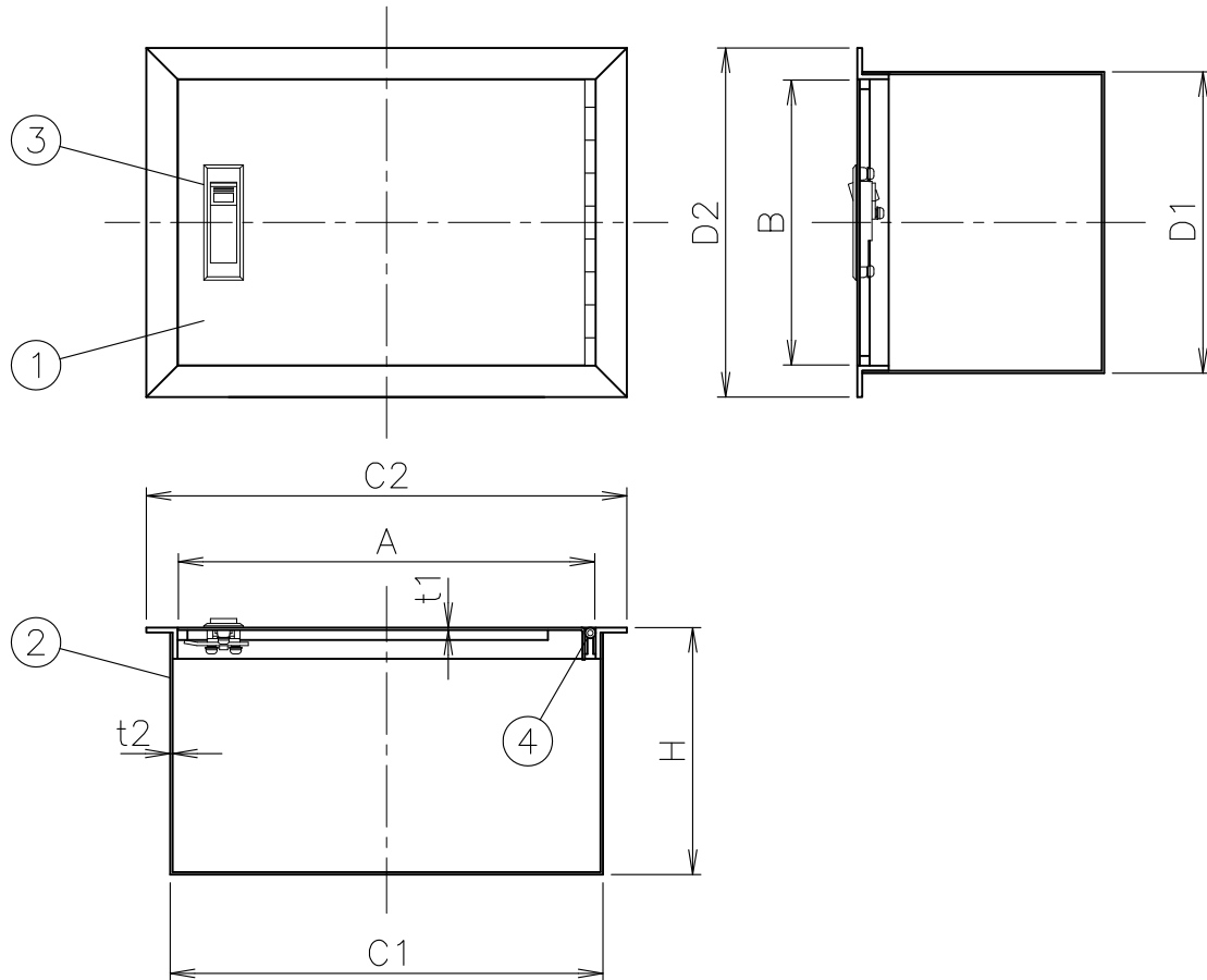
寸法表
