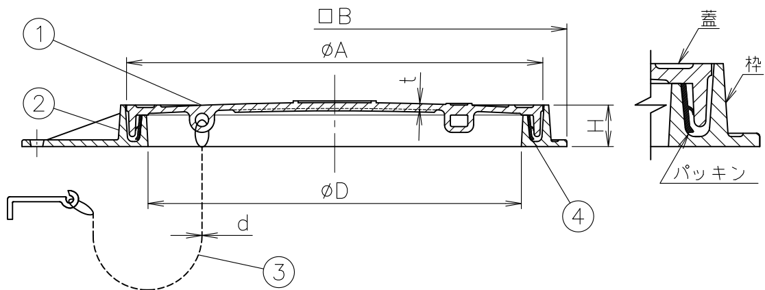
端部詳細
