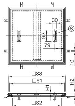
端部詳細
