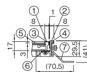
端部詳細
