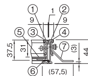
端部詳細
