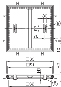
端部詳細
